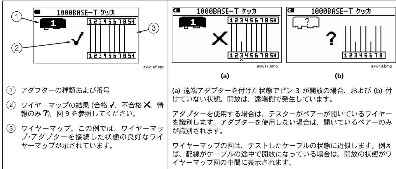
図 10. ワイヤーマップの表示例
